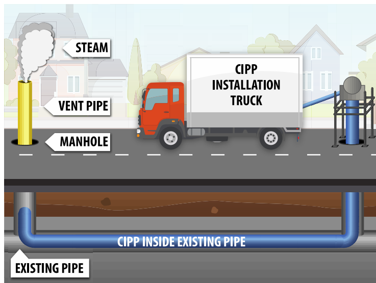
CIPP 安装过程示意图
