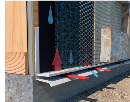
Bottom Vent
